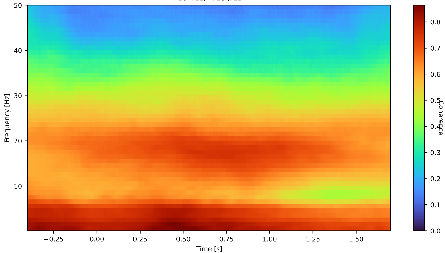
PEC (P11) - PEC (P12)
